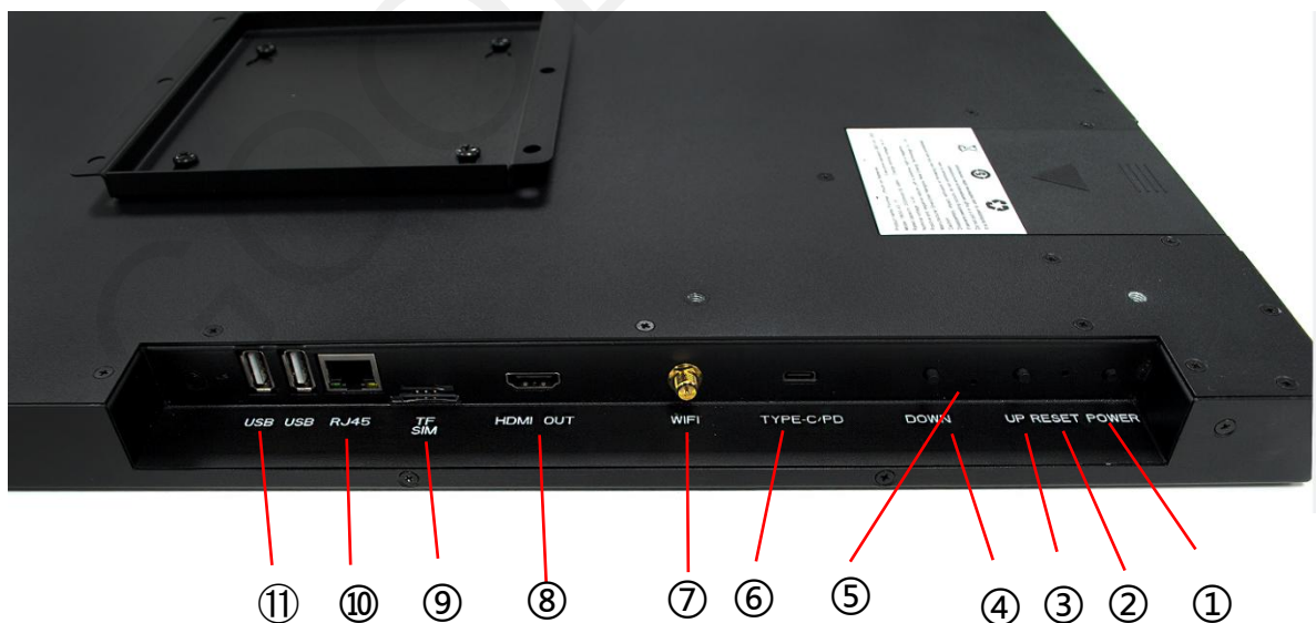
图 3 DMPH253EG1侧面图
