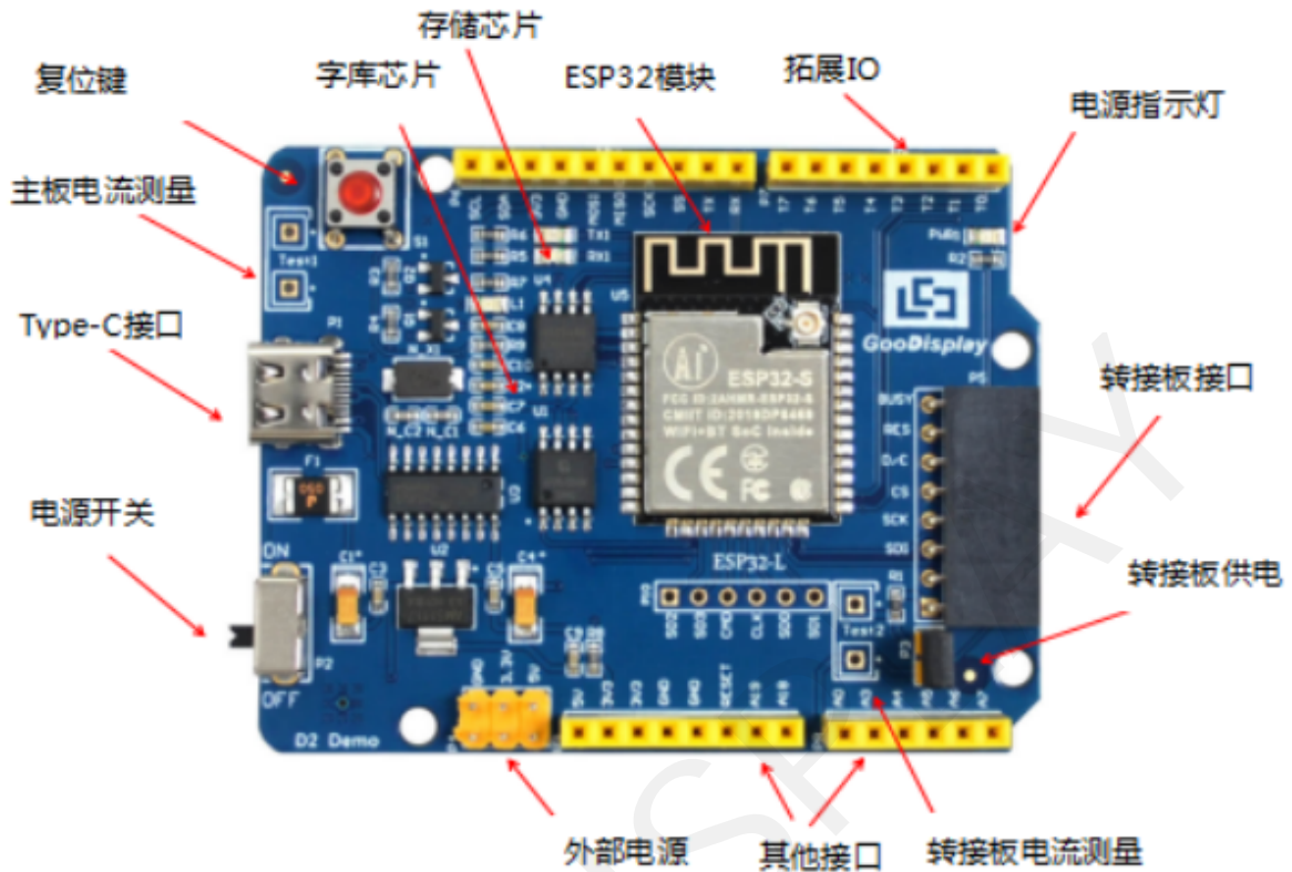
图 1 主板 DESPI-M02L 功能图
