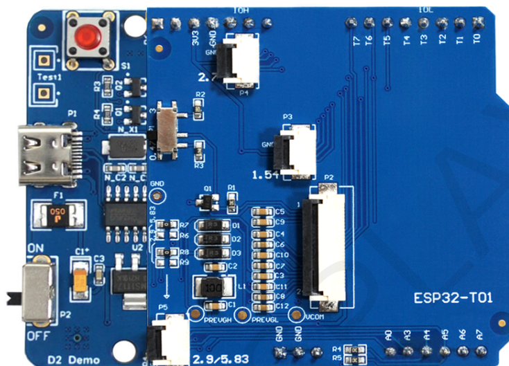
图 3 主板与转接板连接方式
