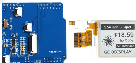
图4 电子纸显示屏与转接板插接示意图
