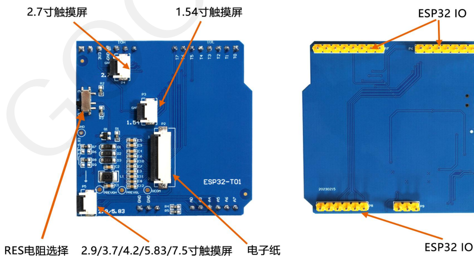
图 2 转接板 ESP32-T01 功能图
